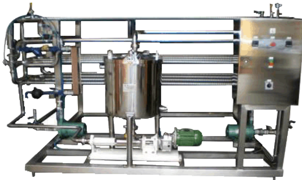
Figura 5. Exemplo de Pasteurizador tipo tubular.
