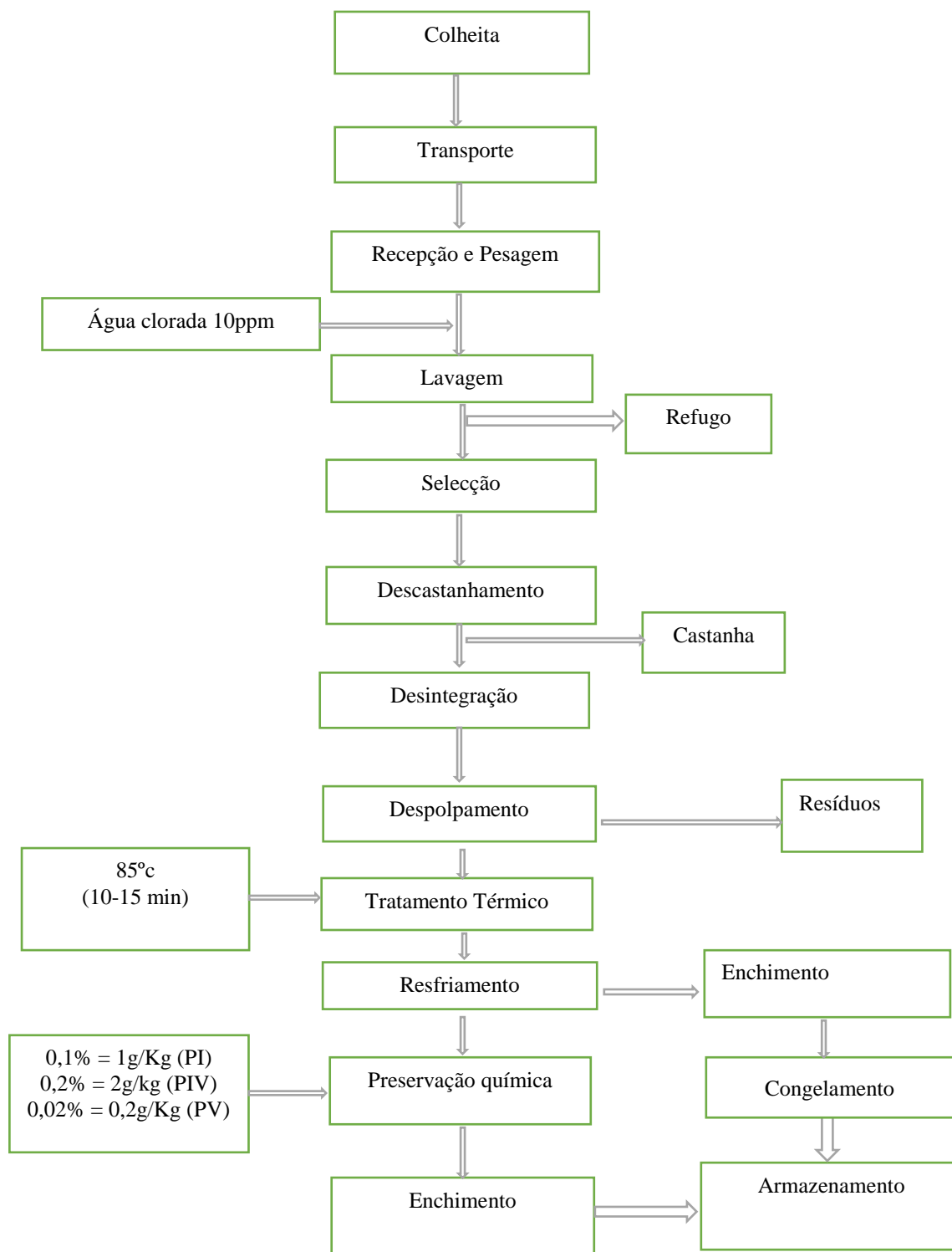
Figura 3. Etapas do processo de produção de polpa de cajú conservada por congelamento e preservada quimicamente.
